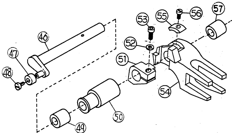
上送り機構 TOP FEED MECHANISM
